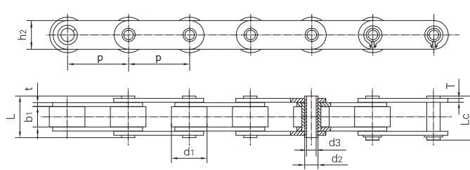
滚子型 ROLLER TYPE(R)
