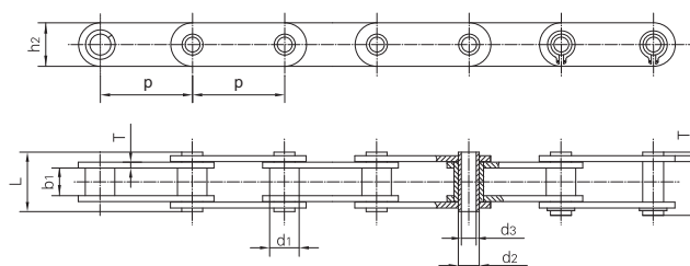
套筒型 BUSHED TYPE(B)
